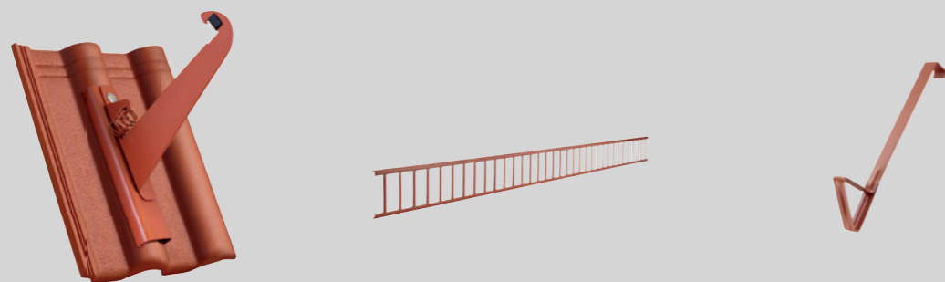
Nosná škridla s držiakom protisnehovej mreže, nutná inštalácia podpornej laty
