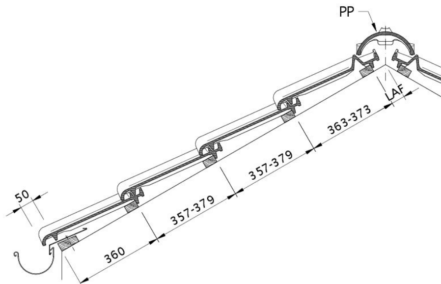
Technický výkres škridla PREMION DQF DQF
